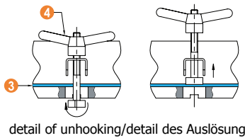
detail of unhooking/detail des Auslösung
